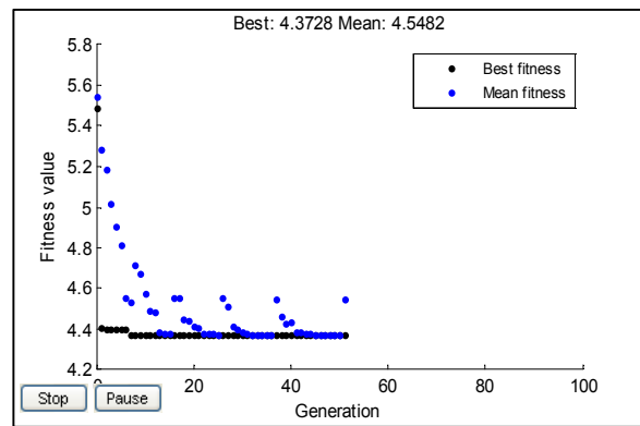
الشكل (2) : يبين علاقة عدد الأجيال المتولدة مع دالة الهدف ( الفقد بالقدرة الحقيقية عند الإضافة لموقع واحد )
